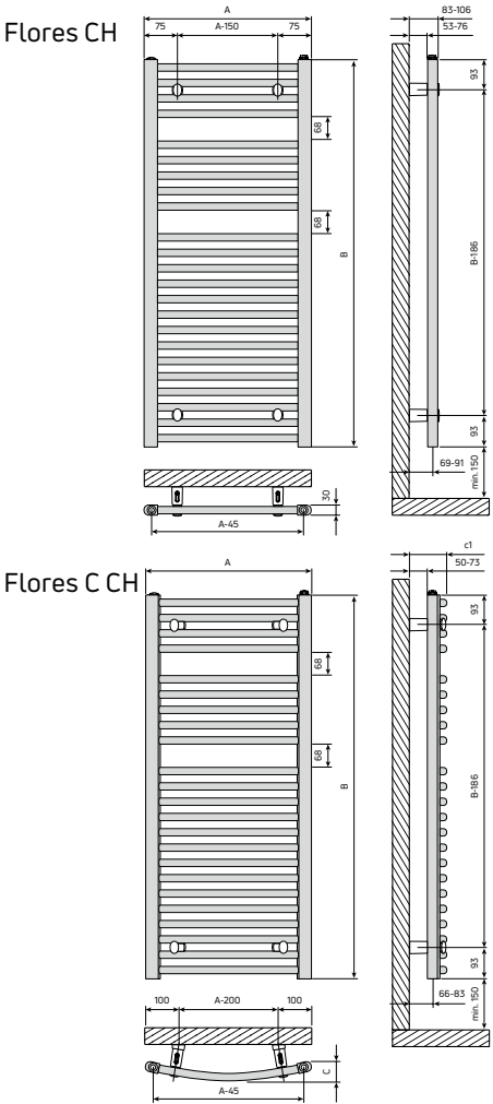
Abb. 73 Badheizkörper Flores CH (links) und Flores C CH (rechts)
