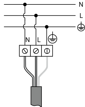
Abb. 61 Elektrischer Anschluss
