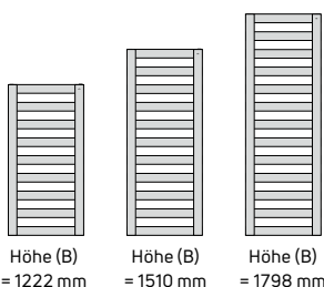
Abb. 18 Rohranordnung
