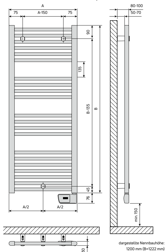
Abb. 108 Abmessungen und Montage Maße
