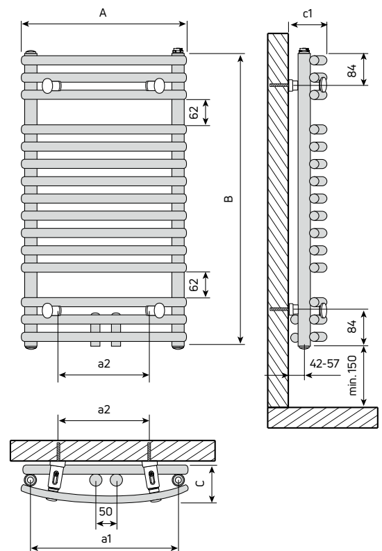
Abb. 80 Badheizkörper Santorini CM
