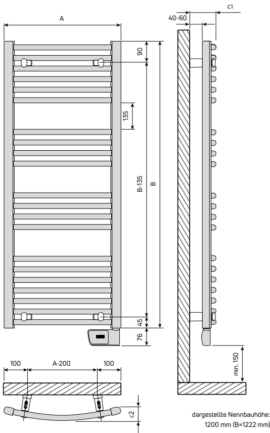
Abb. 111 Rein elektrischer Badheizkörper Flores C E
