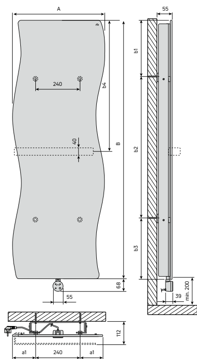
Abb. 36 Design-Badheizkörper Impulse E
