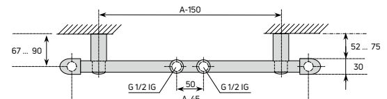
Abb. 68 Anschlussabstände Flores M
