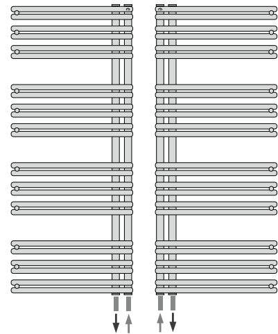
Abb. 8 Anschluss
