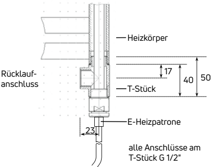
Abb. 115 Montage der PTC-Heizpatrone mit T-Stück an Heizkörpern ohne Anschluss mit 50 mm Nabenabstand (Flores und Flores C)
