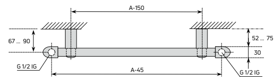
Abb. 67 Anschlussabstände Flores
