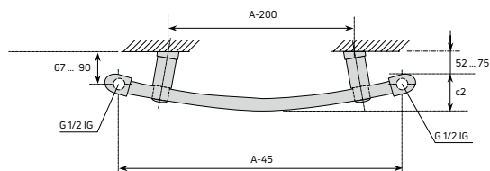
Abb. 71 Anschlussabstände Flores C
