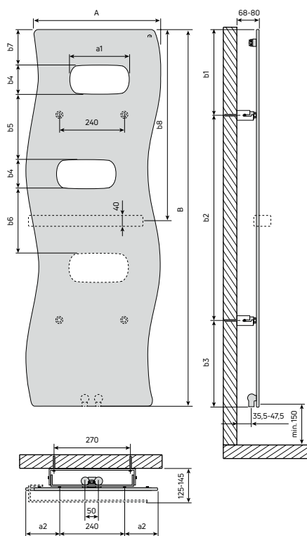
Abb. 33 Design-Badheizkörper Impulse
