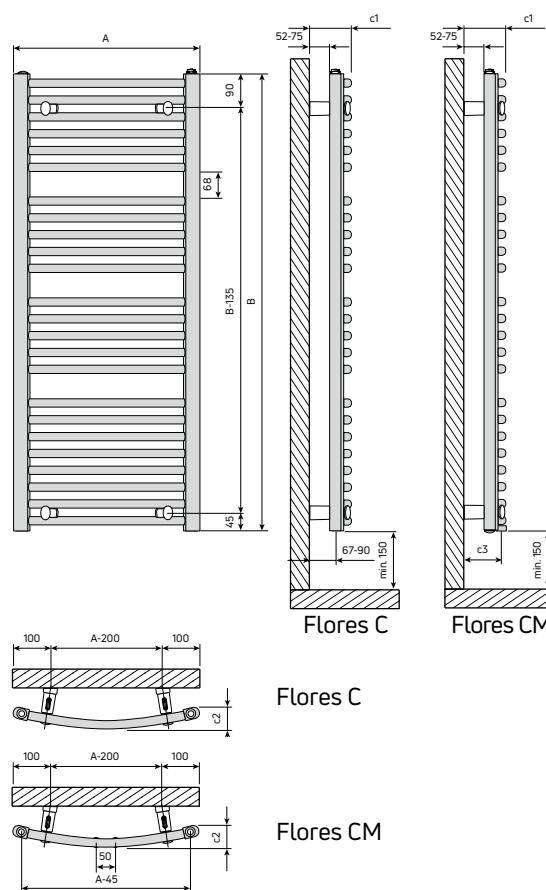
Abb. 69 Badheizkörper Flores C
