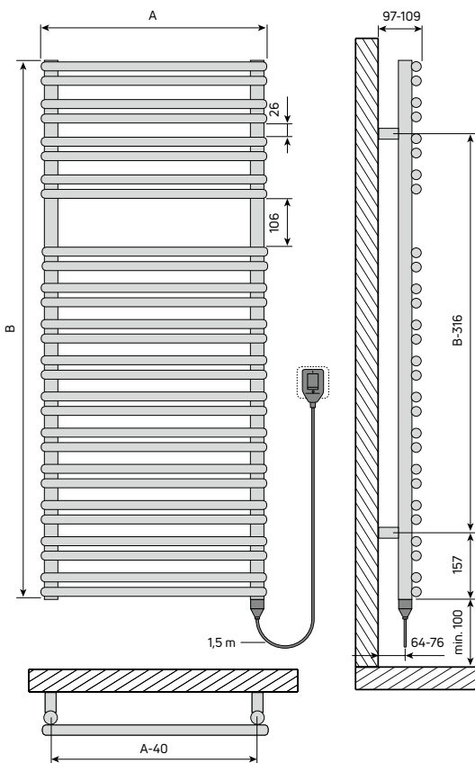
Abb. 106 Abmessungen und Montage Maße
