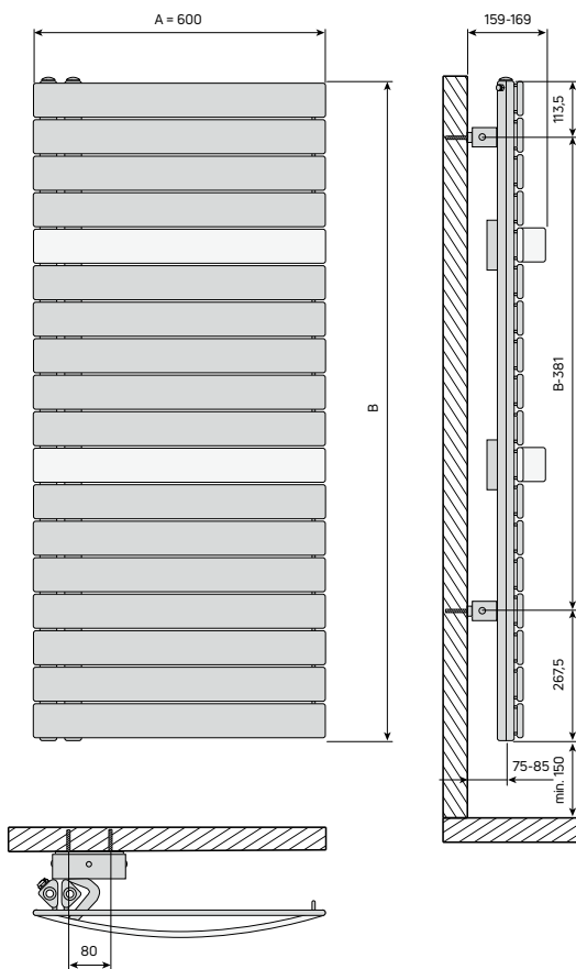
Abb. 93 Abmessungen und Montage Maße (Darstellung: Anschluss links = Standard)
