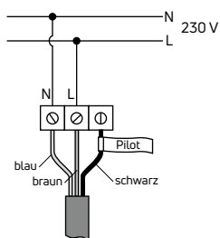
Abb. 109 Elektrischer Anschluss
