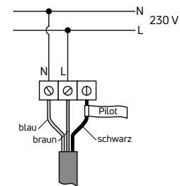
Abb. 98 Elektrischer Anschluss
