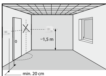
Abb. 101 Abmessungen und Montage Maße
