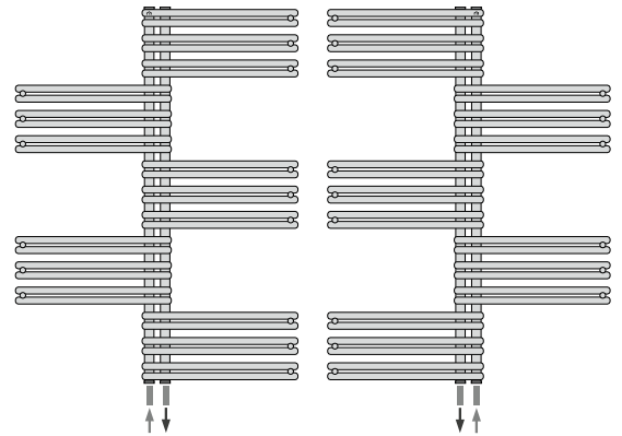
Abb. 22 Anschluss
