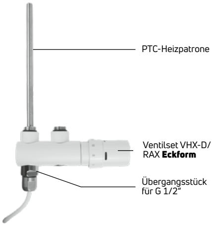
Abb. 116 Montage der PTC-Heizpatrone in Verbindung mit Ventilset VHX-D / RAX Eckform und Übergangsstück für Twist, Gate, Elato, Apolima und Evia
