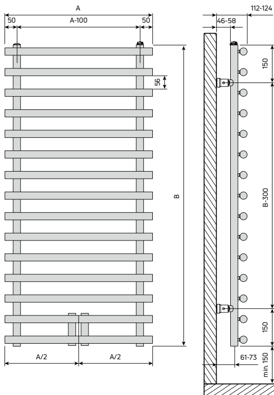
Abb. 84 Badheizkörper Leros
