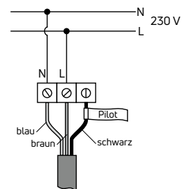
Abb. 113 Elektrischer Anschluss
