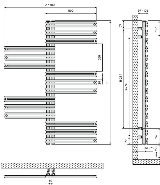
Abb. 20 Abmessungen und Montage Maße
