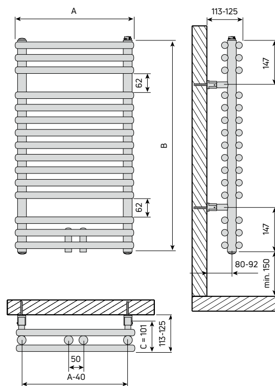
Abb. 83 Abmessungen und Montage Maße
