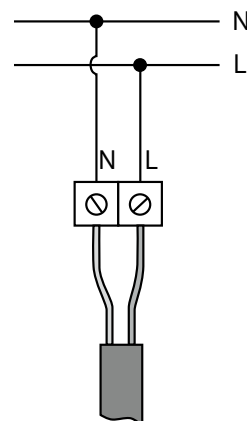
Abb. 64 Elektrischer Anschluss
