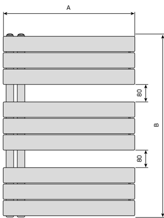
Abb. 89 Badheizkörper Elato
