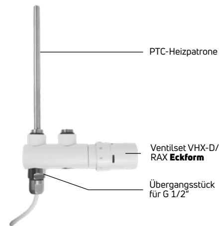
Abb. 116 Montage der PTC-Heizpatrone in Verbindung mit Ventilset VHX-D / RAX Eckform und Übergangsstück für Twist, Gate, Elato, Apolima und Evia
