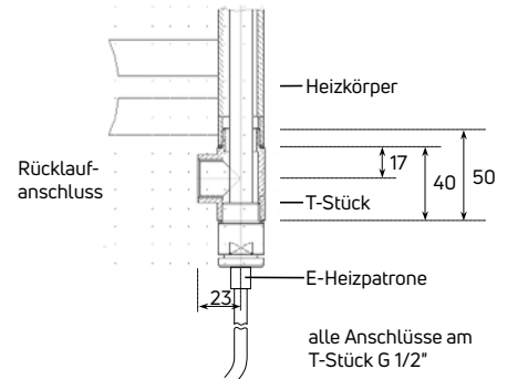
Abb. 115 Montage der PTC-Heizpatrone mit T-Stück an Heizkörpern ohne Anschluss mit 50 mm Nabenabstand (Flores und Flores C)
