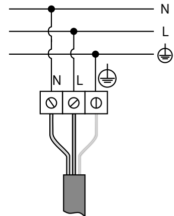
Abb. 61 Elektrischer Anschluss
