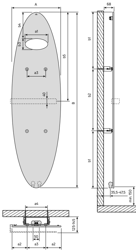
Abb. 27 Design-Badheizkörper Ellipse
