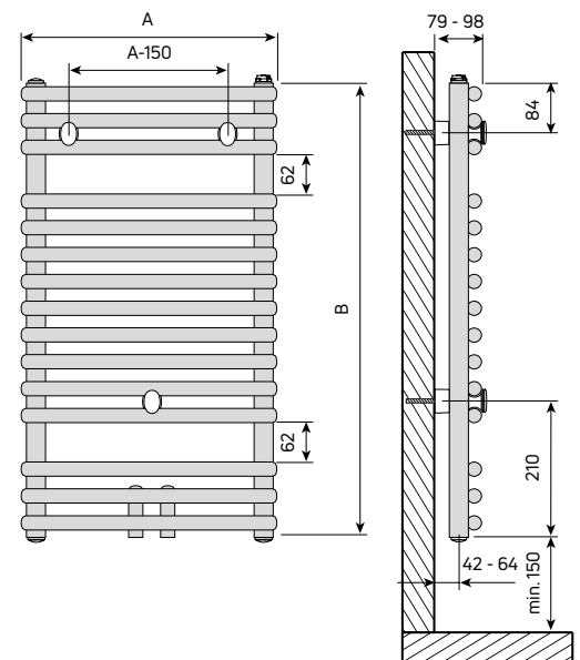
Abb. 78 Badheizkörper Santorini M
