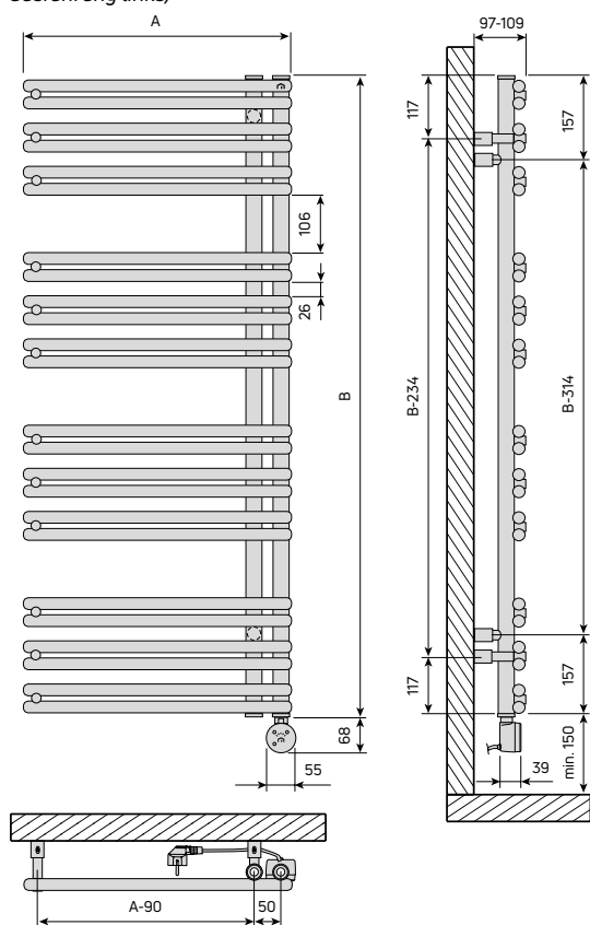
Abb. 10 Abmessungen und Montagemaß
