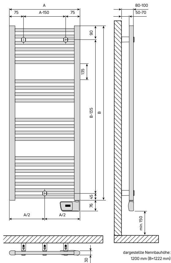
Abb. 108 Abmessungen und Montagegröße
