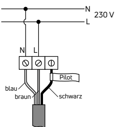
Abb. 109 Elektrischer Anschluss
