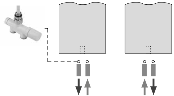
Abb. 57 Anschluss
