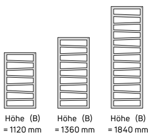
Abb. 45 Rohranordnung
