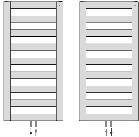
Abb. 15 Anschluss
