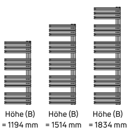
Abb. 10 Abmessungen und Montagemaß
