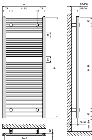
Abb. 73 Badheizkörper Flores CH (links) und Flores C CH (rechts)
