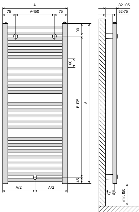
Abb. 65 Badheizkörper Flores M
