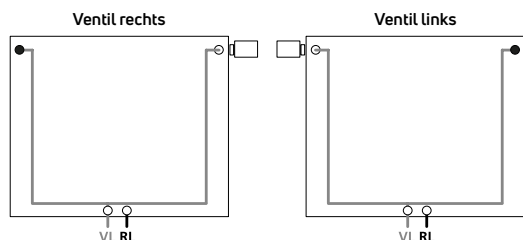
Abb. 41 Anschlusslage Ventil rechts oder Ventil links durch Ventilwechselfunktion (VL=Vortlauf, RL=Rücklauf, Vortlauf immer links!)
