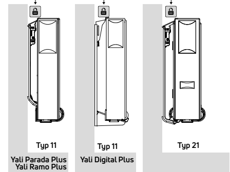
Abb. 90 Die FZ-Halterungen verfügen über eine integrierte Aushebesicherung. Diese ist jeweils nach erfolgter Montage gemäß Abbildung zu aktivieren.
