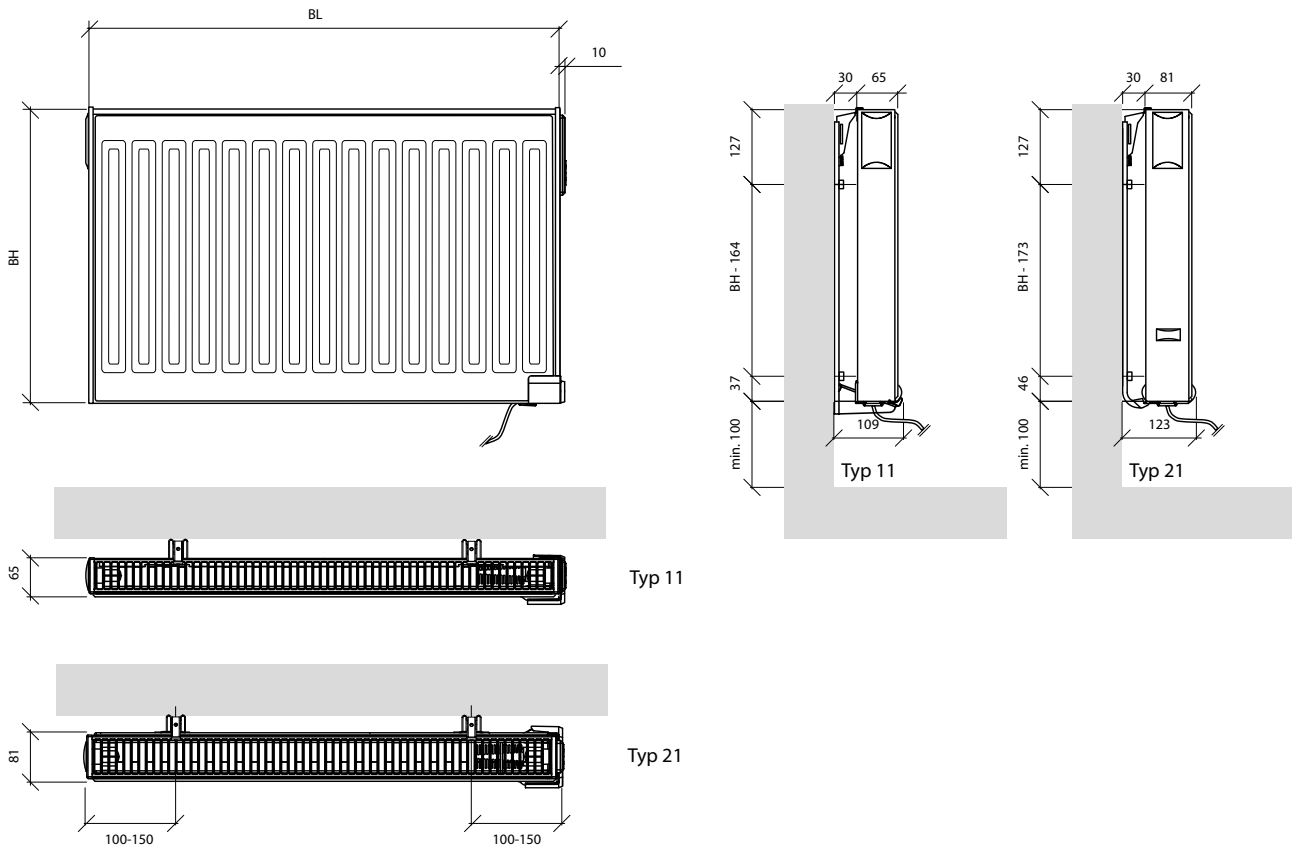
Abb. 102 Montage Maße Yali Digital Plus
