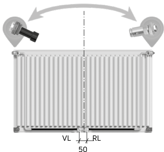
Abb. 45 Integrierte Ventilgarnitur für den Mittenanschluss mit Ventilwechselfunktion. Schnitt und Funktionsmaße (in mm, VL=Vorlauf, RL=Rücklauf)
