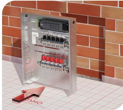
1. Einbau des Fertigverteilerschränkes an gewünschte Wandposition
